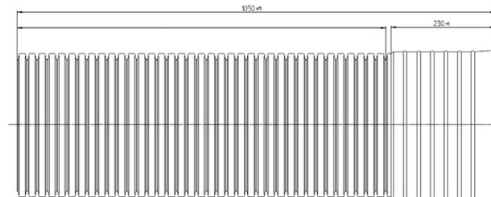
Figure 11 : Rehausse
