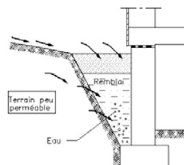
Figure 3 : Accumulation d'eau en pied de fondation
