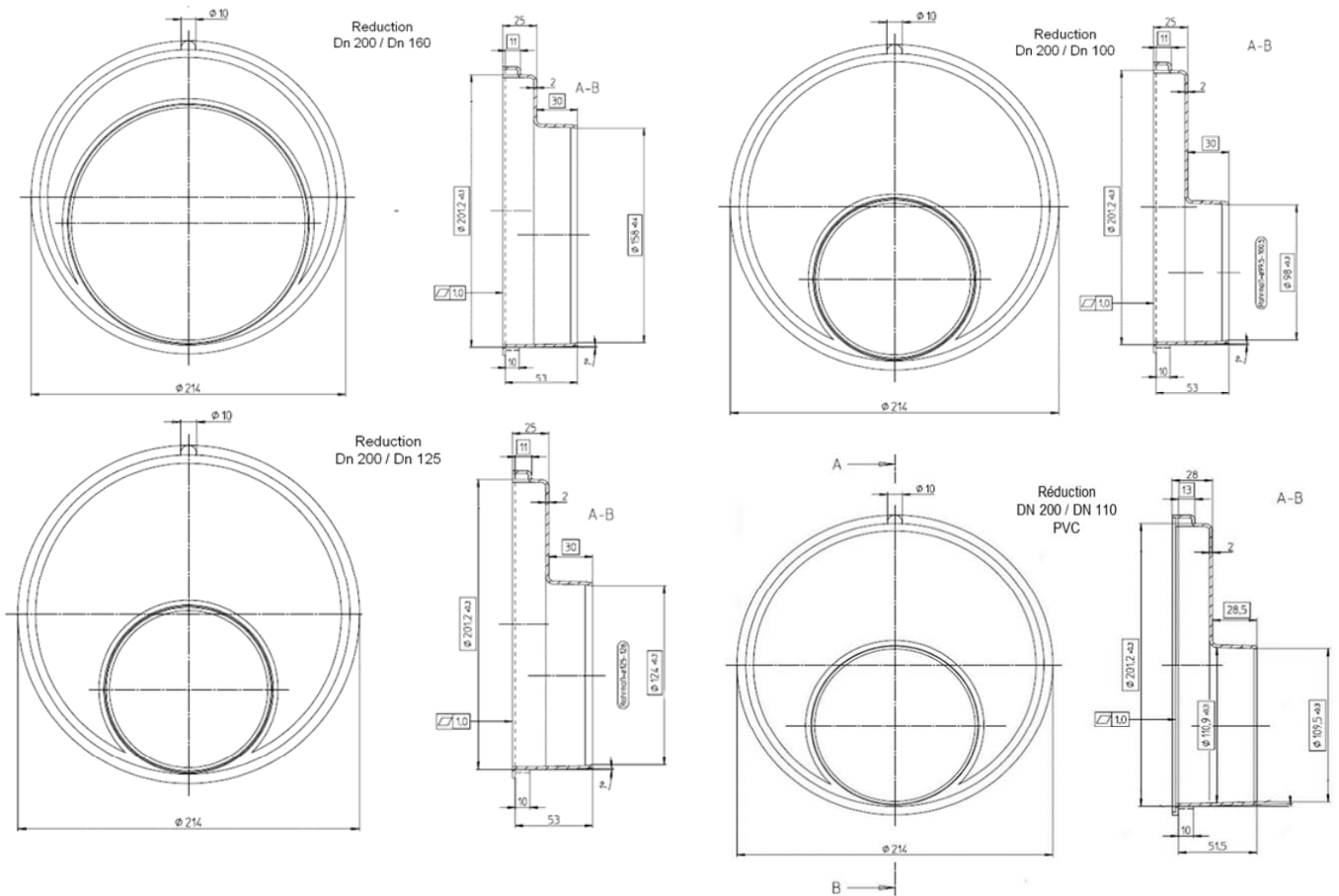
Figure 16 : Pièces de réduction
