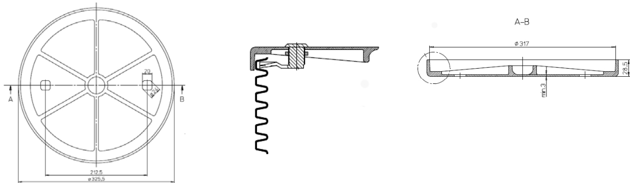
Figure 14 : Couvercle de fermeture en Aluminium
