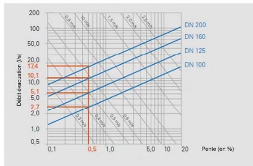
Figure 6 : Choix du diamètre
