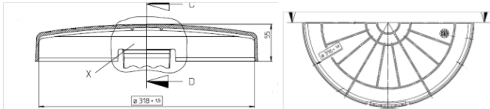
Figure 13 : Couvercle de fermeture en Polypropylène
