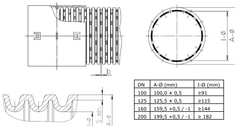
Figure 8 - Caractéristiques dimensionnelles du drain
